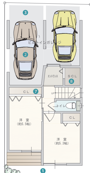
1階平面図
