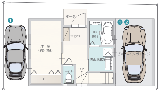
1階平面図
